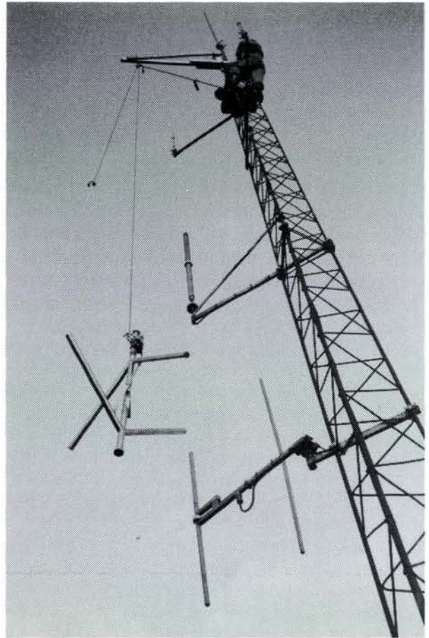
Antenna vert montert på Liafjellet 28. januar 1989. (Foto: Arne Aarseth).
